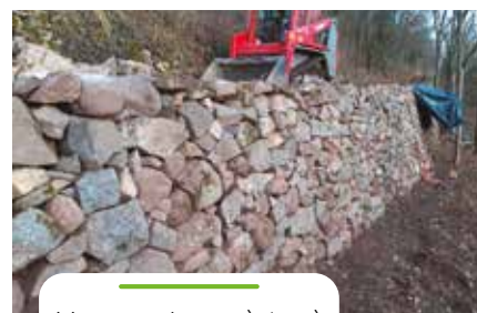
Muret en pierres sèches à Vieux-Thann
